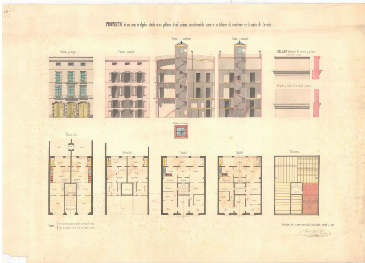
Pujol Salomó, Antonio. Proyecto de una casa de alquiler: fachadas, secciones, plantas y detalles , 1867. AG-000423.
